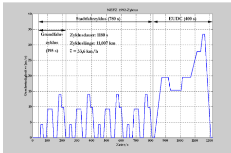
Fahrzyklus
